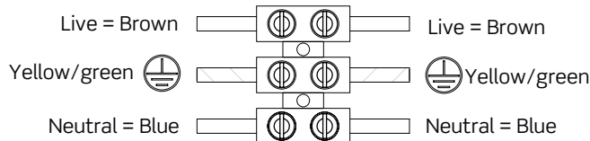
Fig 2. Mains Input
